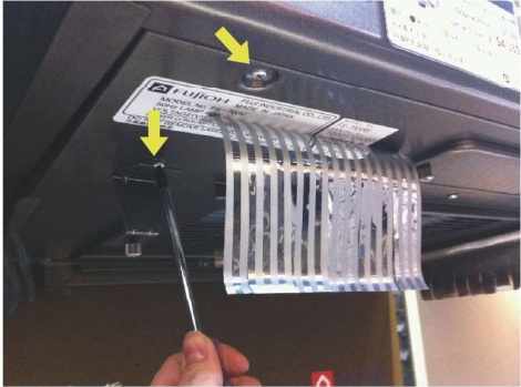
用螺絲批拆除安全保護網的6粒螺絲
